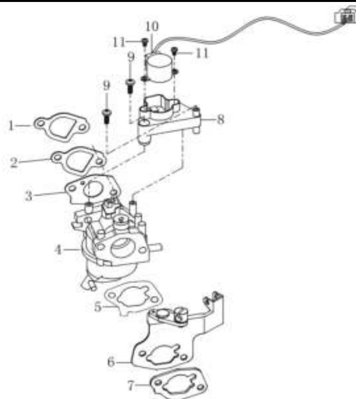
化油器 (CARBURETOR)
